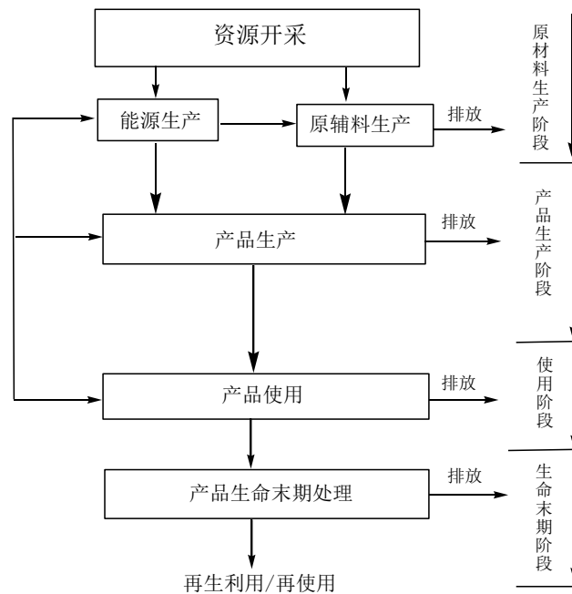
图 B.2 阴极电泳涂料产品生命周期示意图
