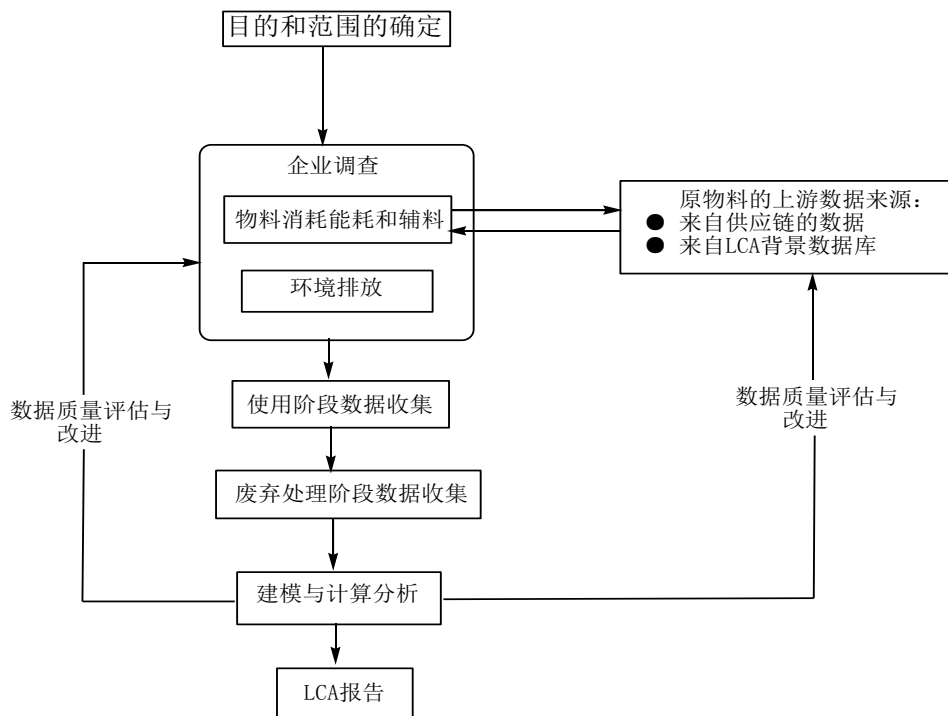
图 B.1 阴极电泳涂料产品生命周期评价基本步骤
