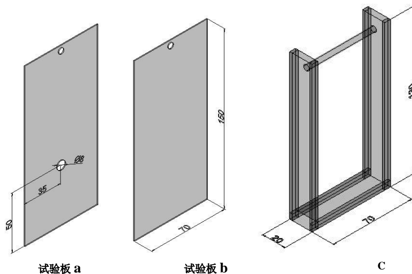
图 A.1 实验用四枚盒板及绝缘框（单位：mm）
